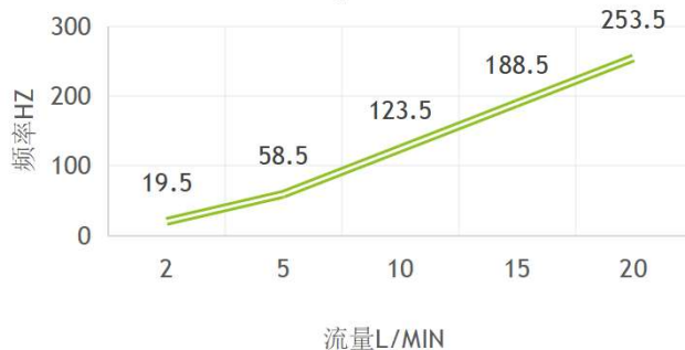
CHLN-01流量与频率曲线 F=13Q-6.5
