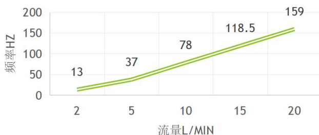
CHLN-01流量与频率曲线 F=8.1Q-3
