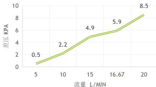
CHEP-02卫浴压差曲线
