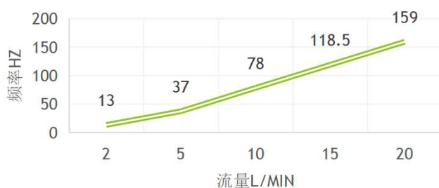
CHIP-02流量与频率曲线 F=8.1Q-3
