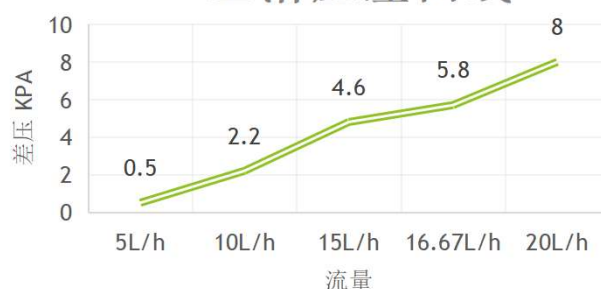
CHEFT-01 卫浴压差曲线
