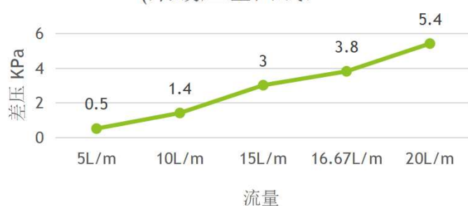
CHMN-07 (采暖压差曲线)
