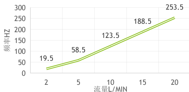
CHI-12流量与频率曲线 F=13Q-6.5
