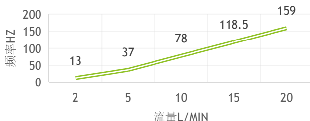
CHI-12流量与频率曲线 F=8.1Q-3
